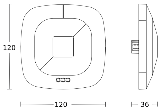
Dessin dimensionnel 1
